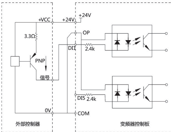
图3-20 源型接线方式
