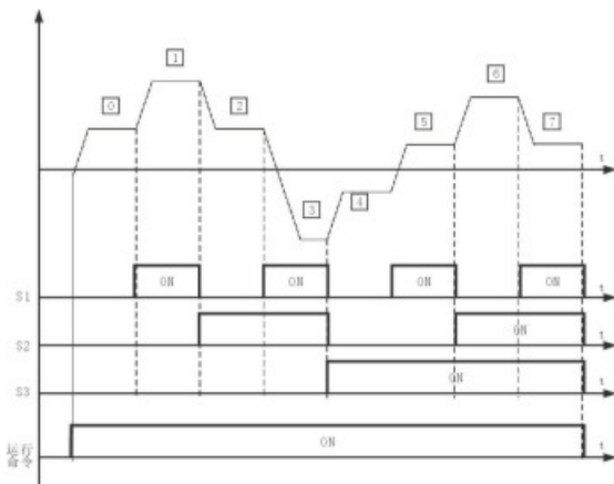
图5-12 多段速度运行逻辑图
