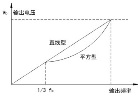
图5-4 V/F曲线示意图
