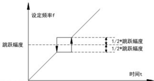
图5-6 跳跃频率示意图
