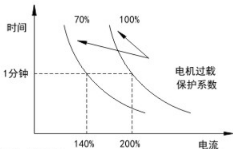
图5-13 电机过载保护系数设定
