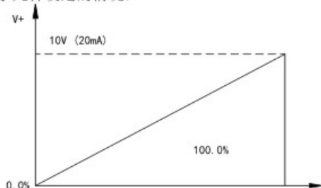
图5-23 给定量与模拟量输出的对应关系
