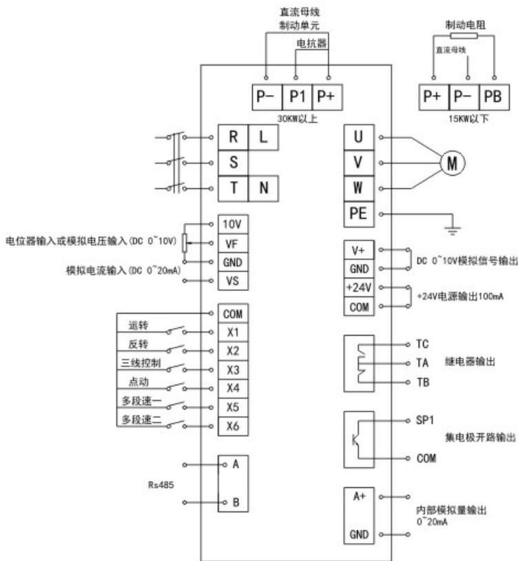
220~460V接线示意图
