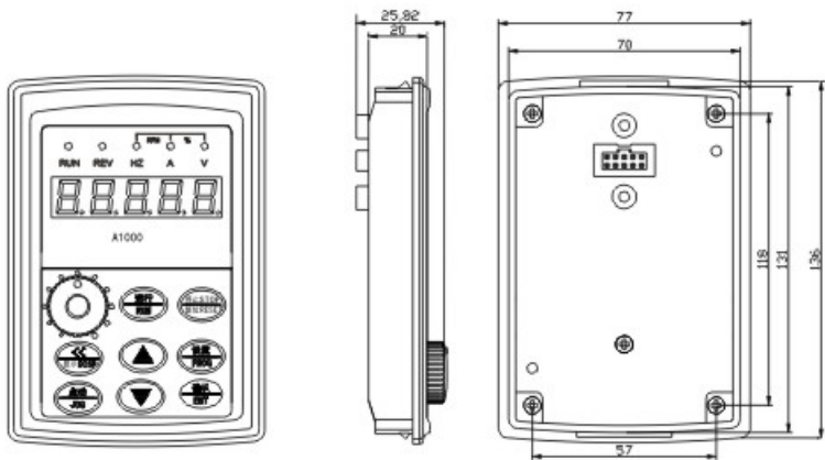
小操作面板安装尺寸
