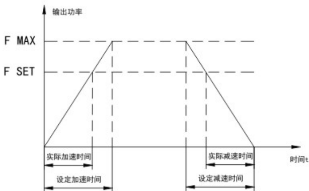
图5-1 加减速时间示意图
