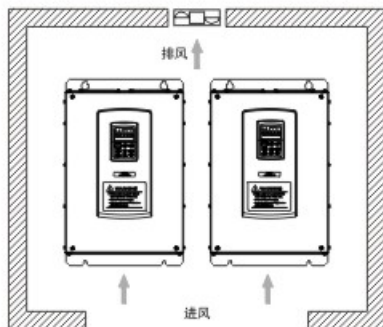
多台壁挂式变频器的安装I
