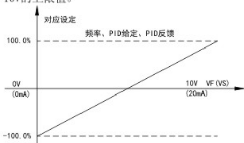
图5-22 模拟给定与设定量的对应关系
