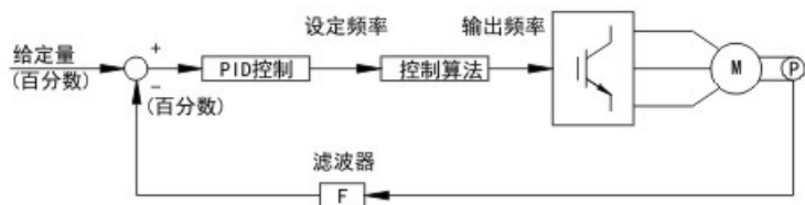
图6-10 过程PID原理框图
