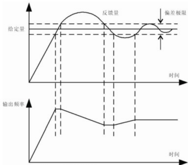
图5-11 偏差极限与输出频率的对应关系
