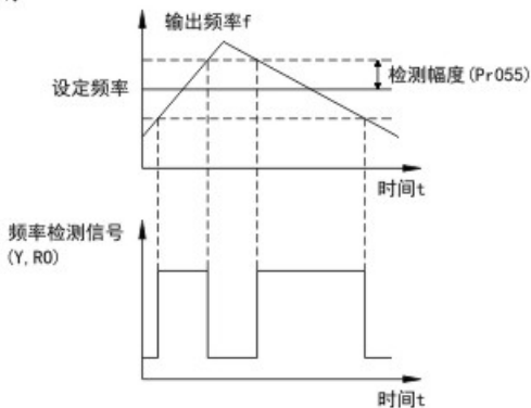
图5-9 频率到达检出幅值示意图
