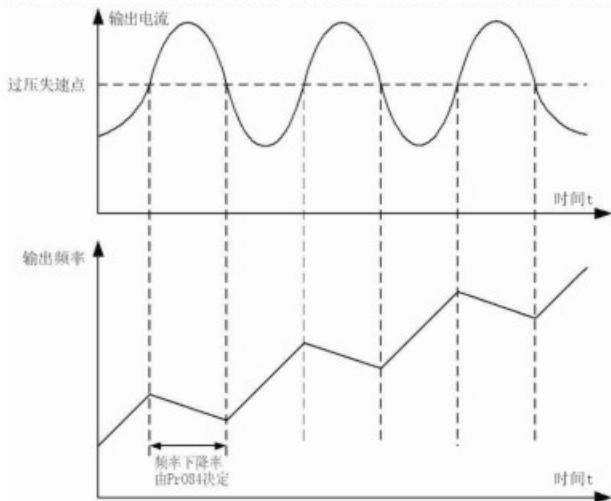
图5-15 限流保护功能示意图
