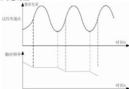
图5-1 过压失速功能
