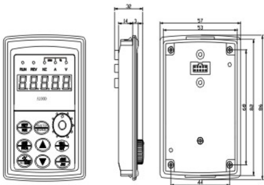
小操作面板安装尺寸
