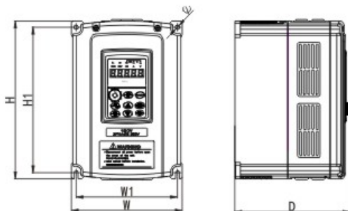
塑壳18.5KW 及以下尺寸
