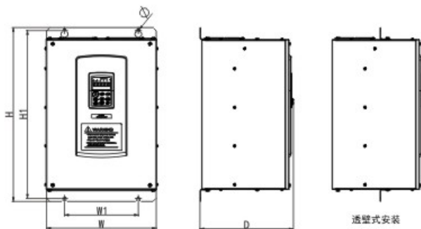
铁壳22KW—132KW（可透壁安装）
