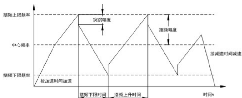
图5-7 摆频运行示意图
