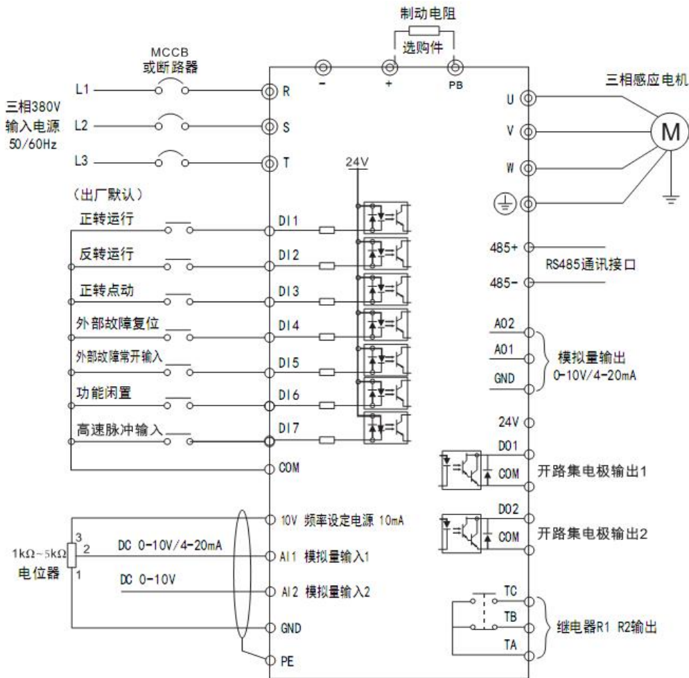
图 4.2 基本运行配线图
