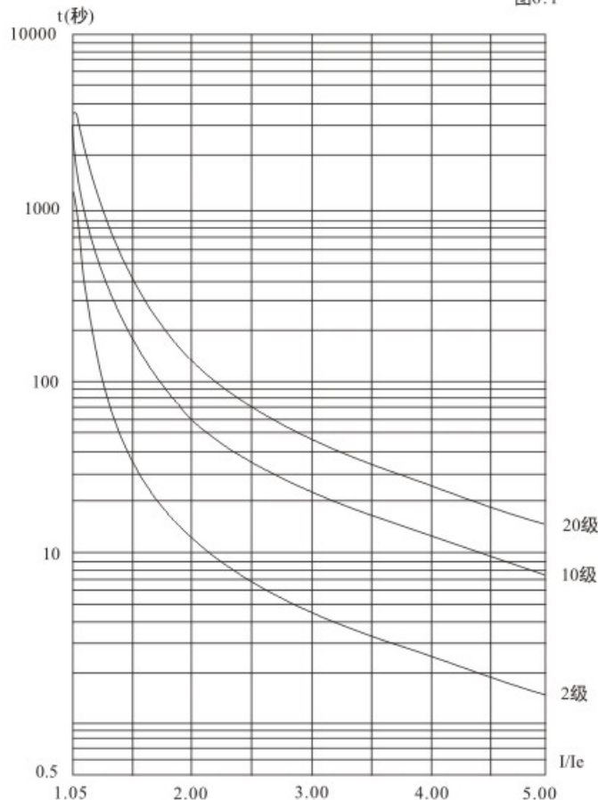
电机热保护脱扣时间曲线(热状态)
